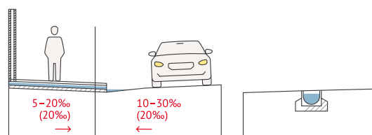
Закрытый лоток
